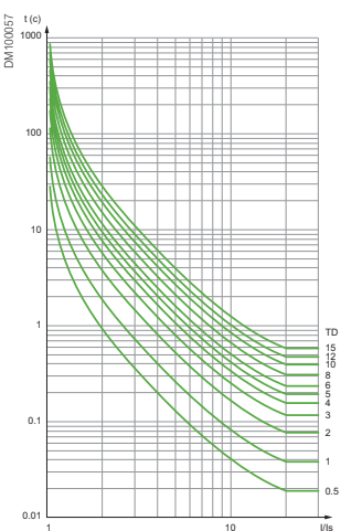
Кривая чрезвычайно обратно-зависимой выдержки времени IEC (IEEE/LI или МЭК/E)
