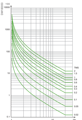
Кривая длительной обратно-зависимой выдержки времени МЭК (МЭК/LT)
