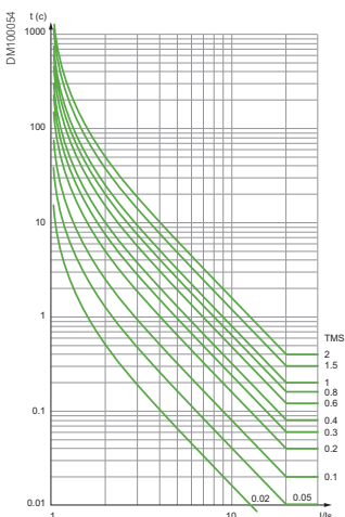
Кривая чрезвычайно обратно-зависимой выдержки времени МЭК (МЭК/ET или МЭК/C)
