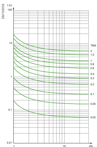
Кривая RI
